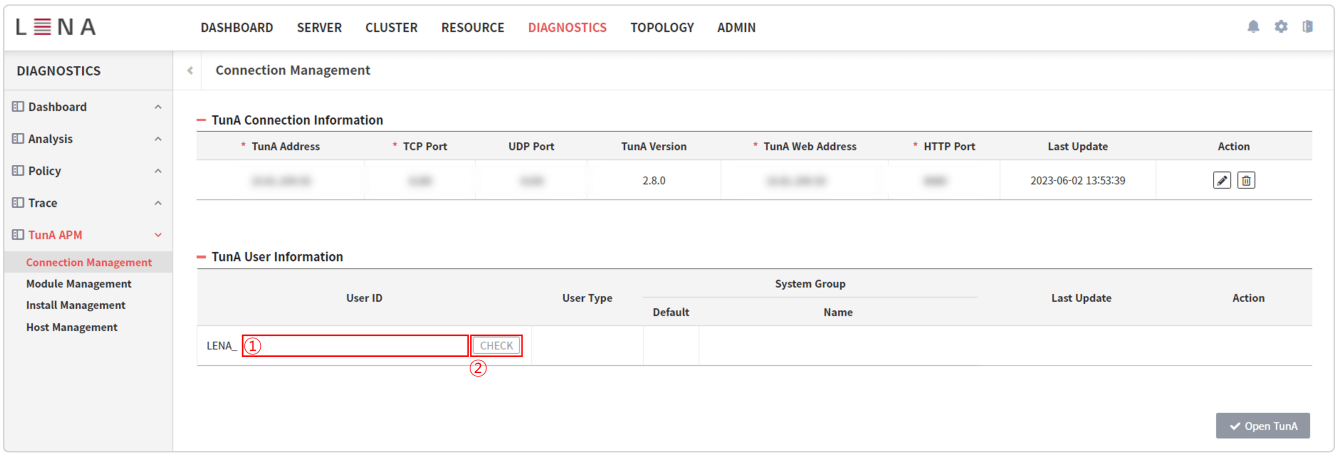
Figure 21. TunA 사용자 정보 입력 화면
