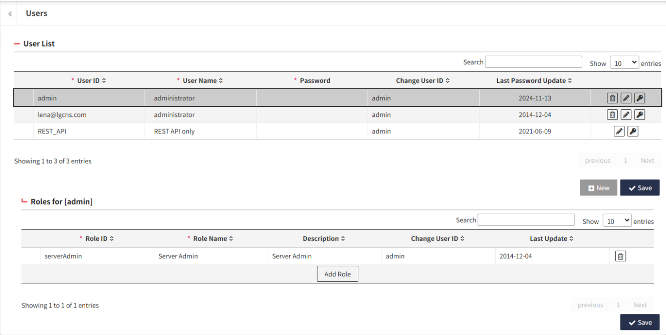
Figure 90. Users 화면
