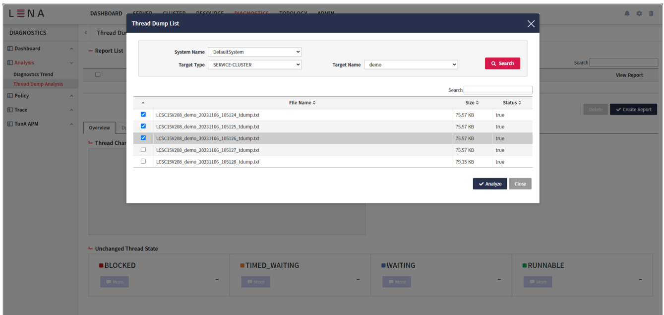
Figure 36. 분석할 Thread Dump를 선택해 Report를 생성하는 모달 창
