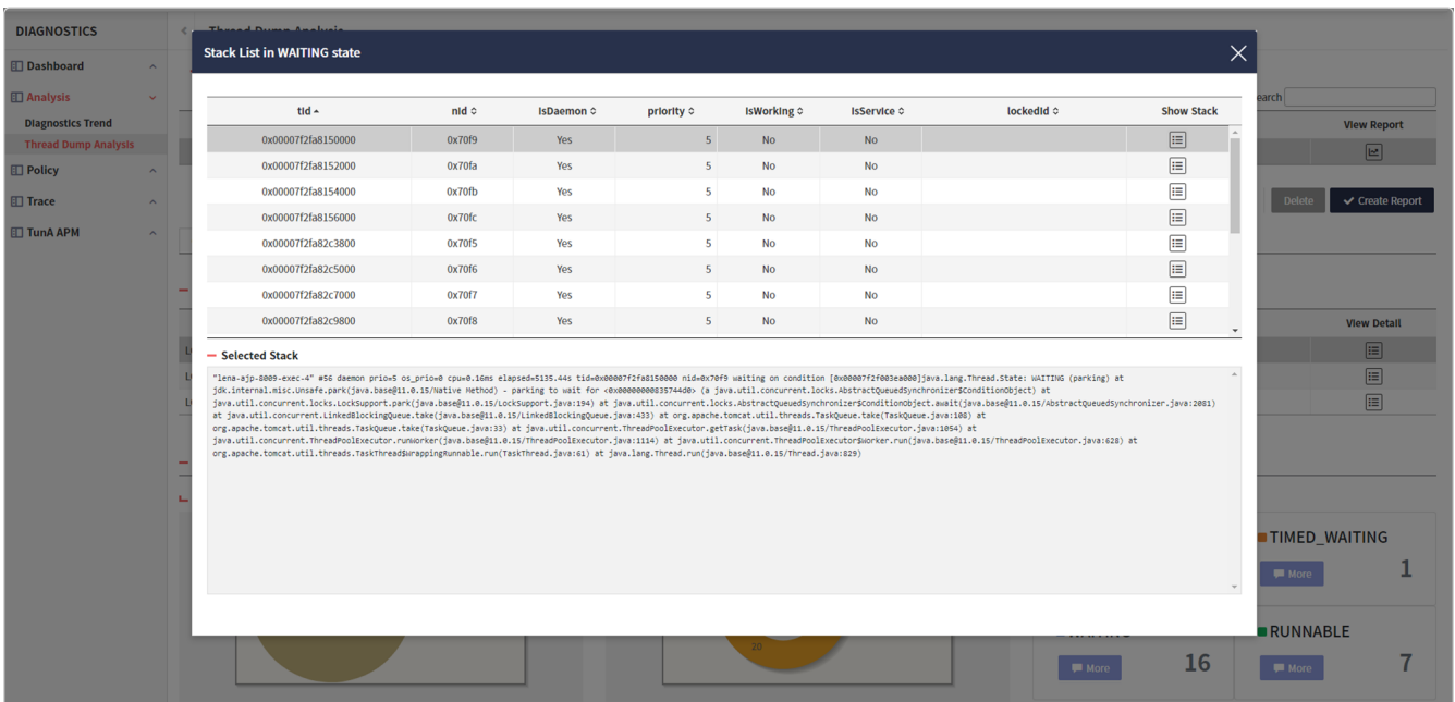
Figure 41. 선택한 Thread Dump 파일 내 상태 별 Thread 정보
