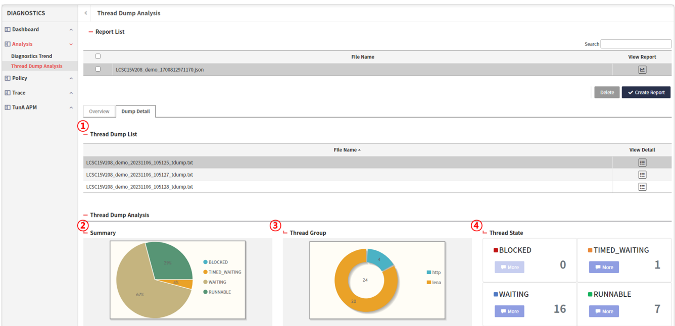
Figure 40. 분석한 Dump 파일 별 Thread 정보를 보여주는 화면
