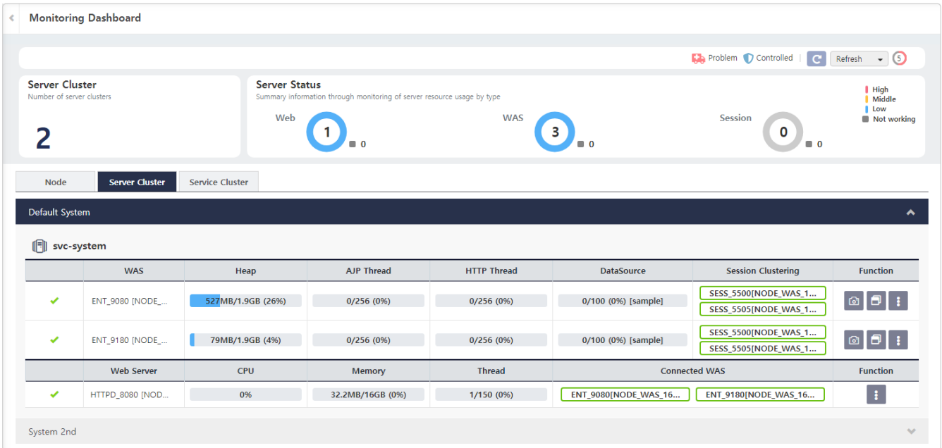
Figure 53. Monitoring Dashboard의 Server Cluster 탭 화면
