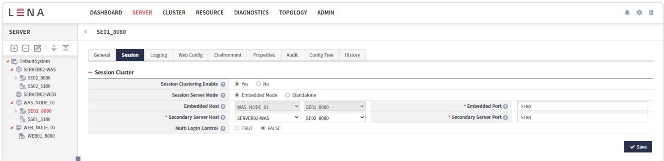
Figure 35. WAS 의 Embedded 모드 Session Server 설정
