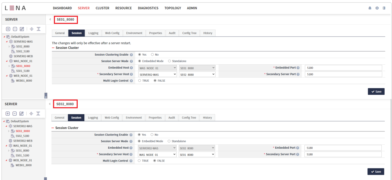
Figure 36. WAS 의 Embedded 모드 Session Server 설정의 완료
