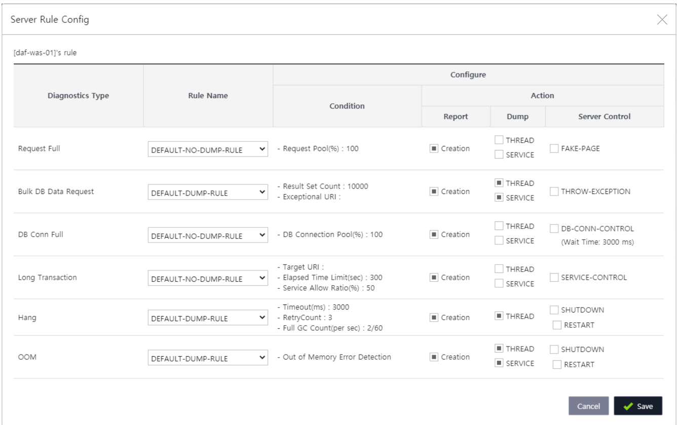
Figure 70. 진단 Rule Mapping 화면
