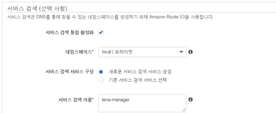
Figure 23. ECS기반 Manager 설치 - Service Discovery 설정
