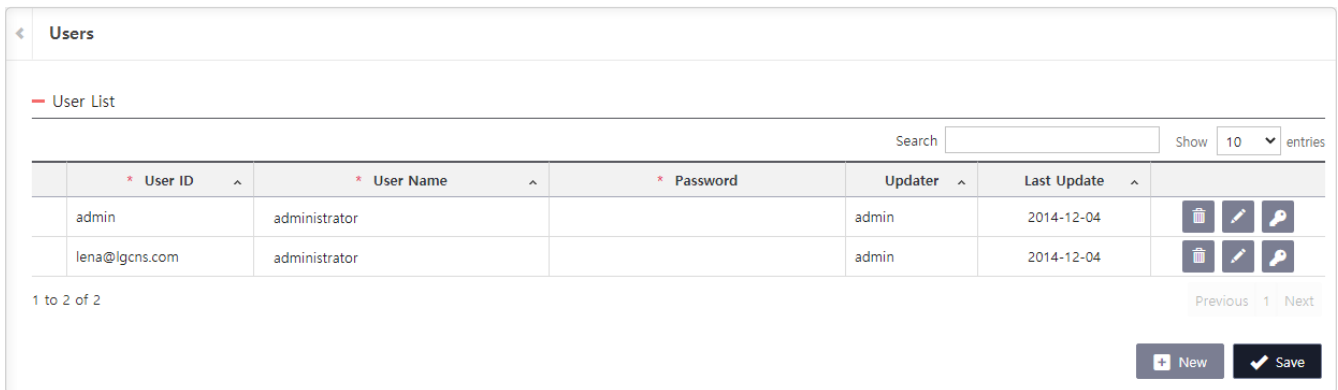
Figure 18. Users 화면
