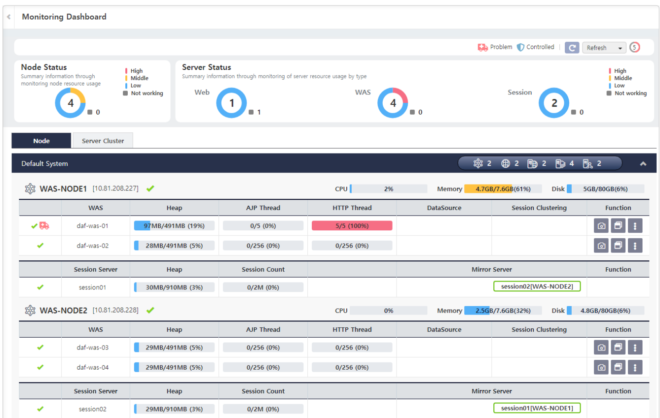
Figure 51. Monitoring Dashboard의 Node 탭 화면
