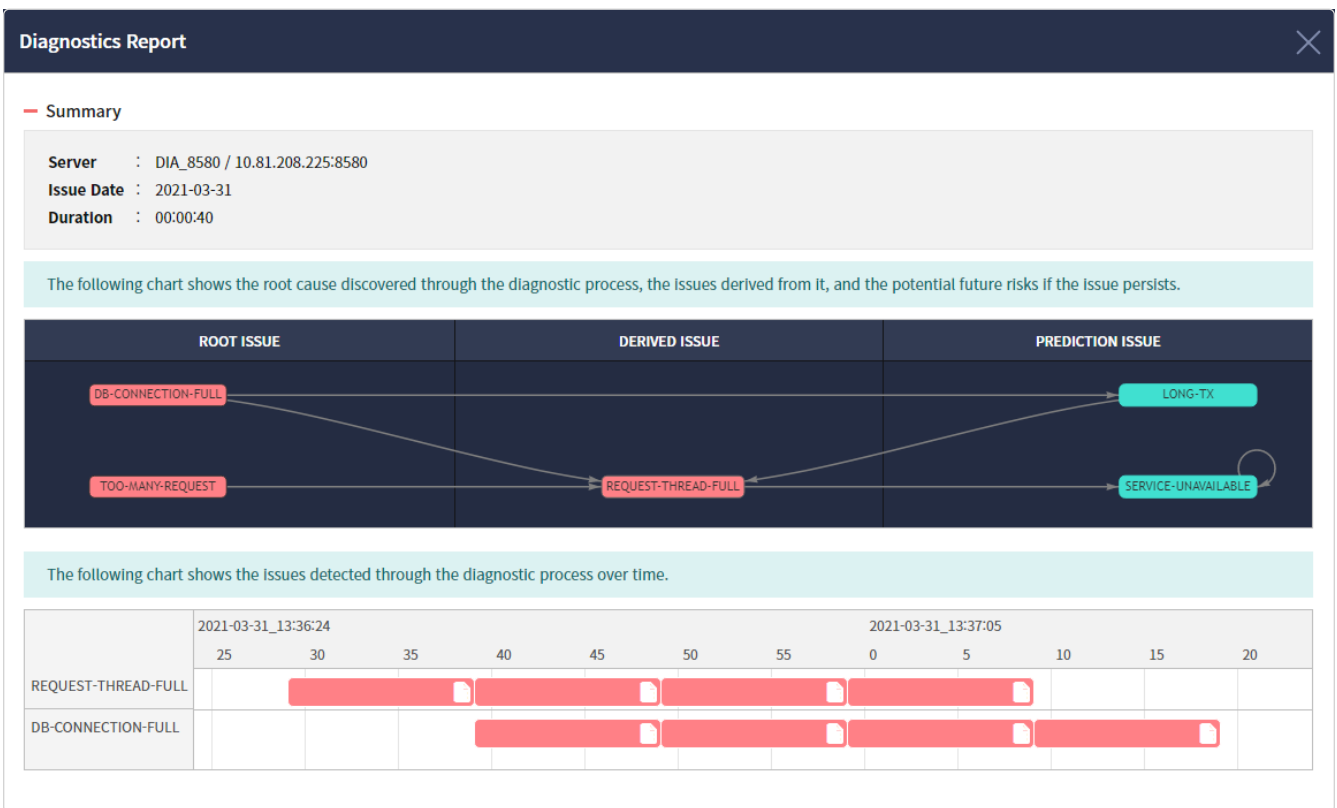
Figure 64. 진단/대응 리포트 화면
